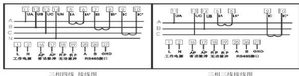
三相四线 接线图
